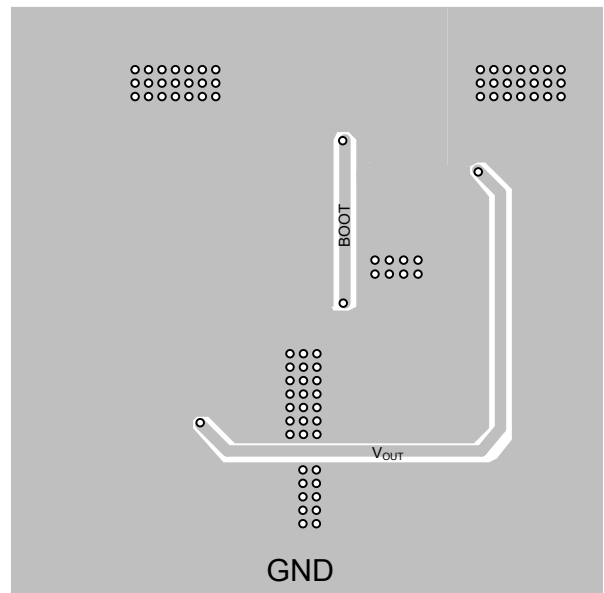
Bottom Layer
