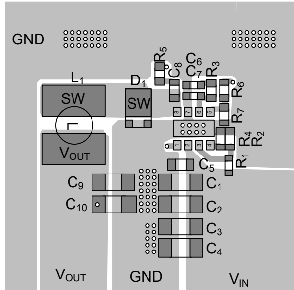
Top Layer
